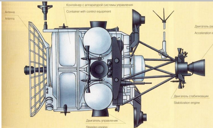
Рис. 14. Космический аппарат ИС
