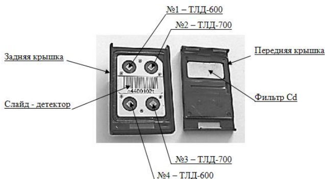
Рис. 6. Конструкция дозиметра 8806
