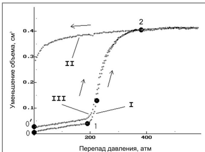
Рис. 1. Зависимость изменения объема от перепада давления.
