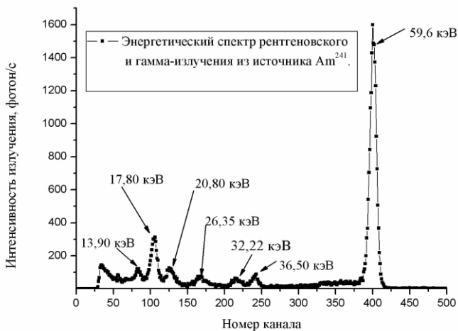
Рис. 4. Измеренный с помощью CdTe-детектора энергетический спектр гамма-излучения из источника \text{Am}^{241}
