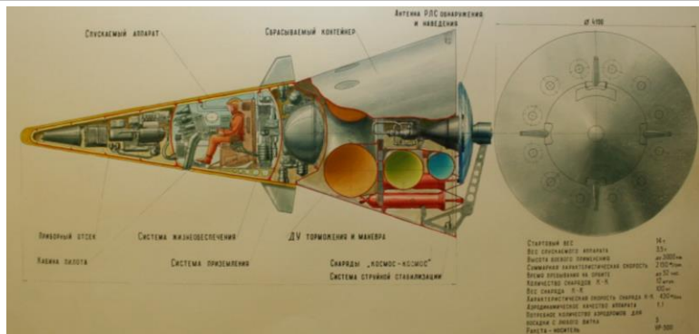
а) Пилотируемый орбитальный истребитель спутников (Схема 4)
