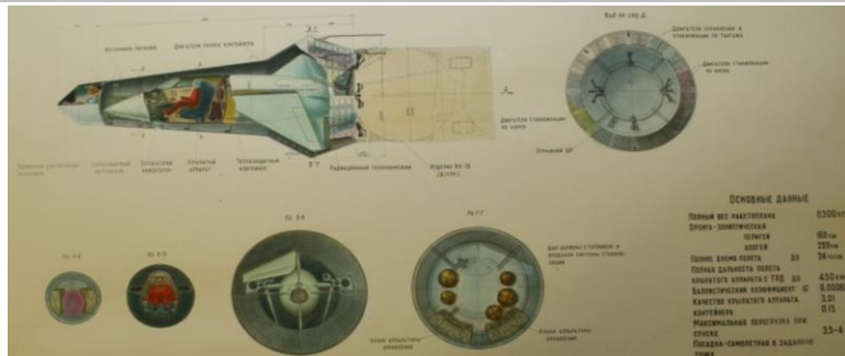
б) Компонентная схема орбитального ракетоплана
