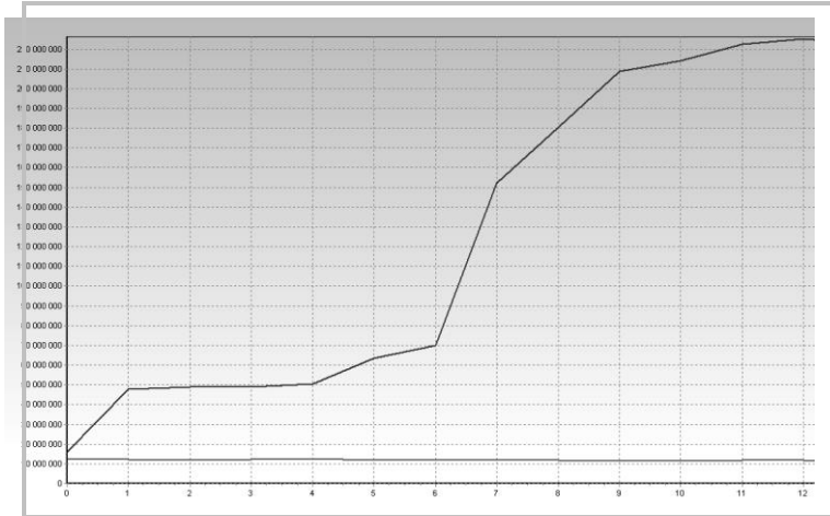
Рис. 1. Сравнение времени поиска минимального значения в списке и массиве (ось абсцисс отражает фрагментацию списка в Кб, ось ординат — количество тактов выполнения шага эксперимента)
